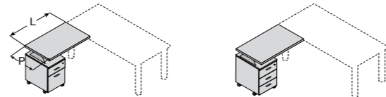
P 60 x H 73,3 L 100 P 60 x H 73,3 L 100
