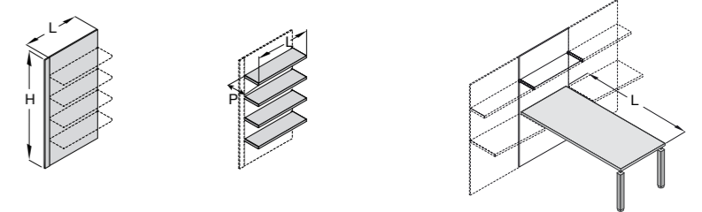
L 45 x H 161,5 L 60 L 90 L 45 x H 201,5 L 60 L 90 L 45,1 x P 27 x H 3,8 L 60,1 L 90,1 L 45,1 x P 49 x H 3,8 L 60,1 L 90,1 P 90 x H 74 L 160 L 180 L 200
