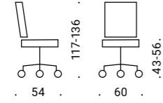
mod. 7139R
