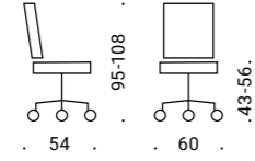
mod. 7539R
