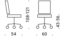
mod. 7531
