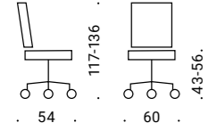
mod. 7131
