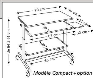
Modèle Compact + option
